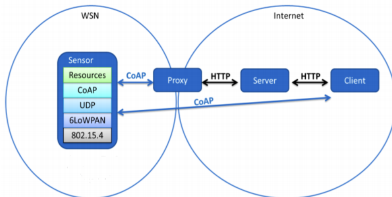
Figura 2.3: Comunicazione COAP
