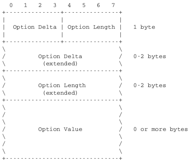
Figura 2.5: Opzioni COAP
