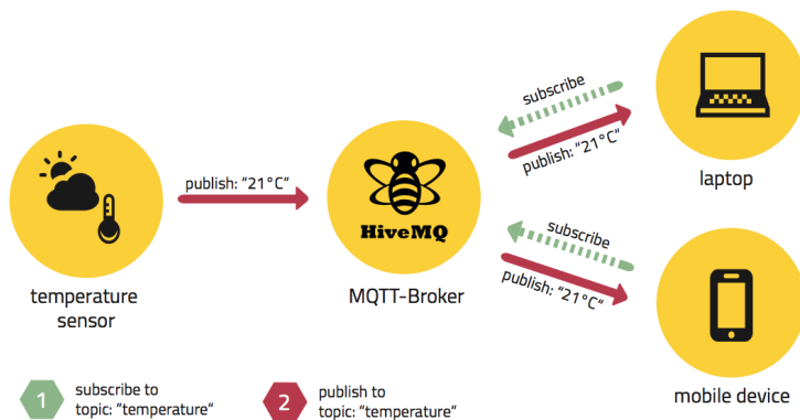
Figura 2.1: Comunicazione MQTT
